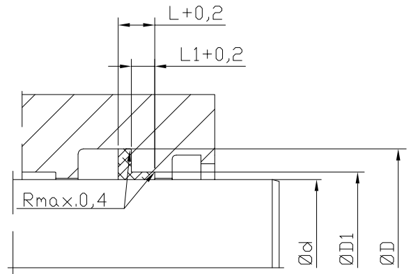
geschlitzte Ausführung
