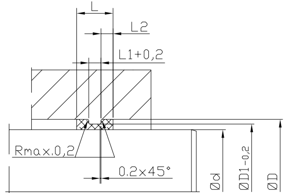
geschlossener Einbauraum
