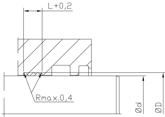
geschlitzte Ausführung
