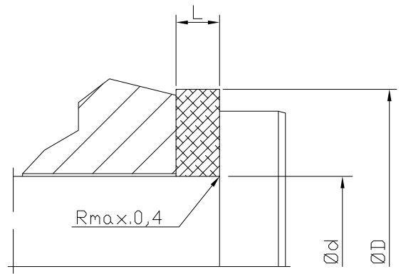
offener Einbauraum
